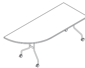
PFT04 2000 / 800 / 740 42.8 kg
